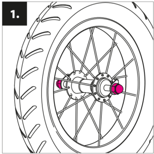
Montage des vorderen Rades: Lockern Sie beide Radmuttern.
